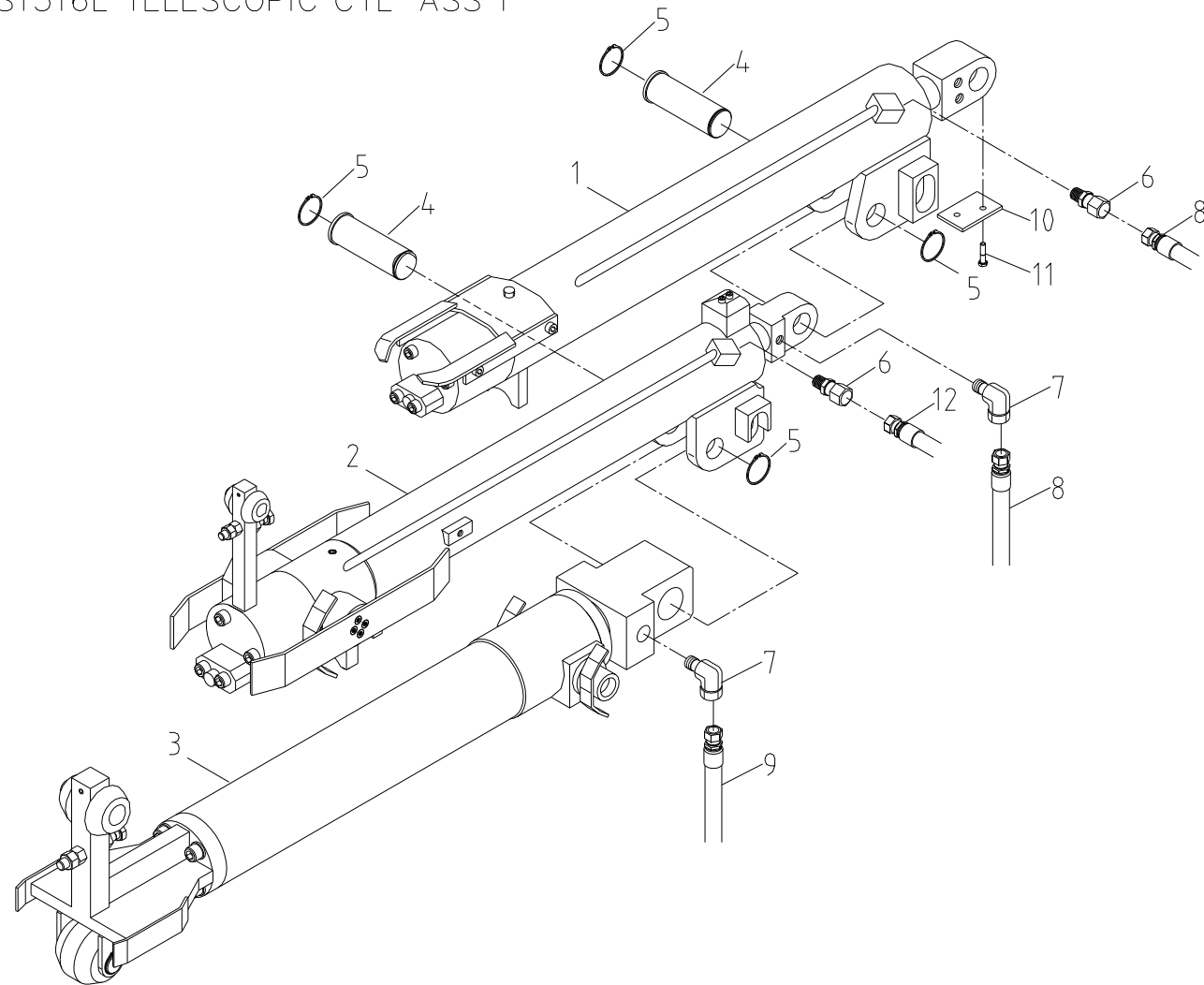
텔레스코픽 실린더 조립체 Fig. 1-1 SCS1516L TELESCOPIC CYL' ASS'Y
