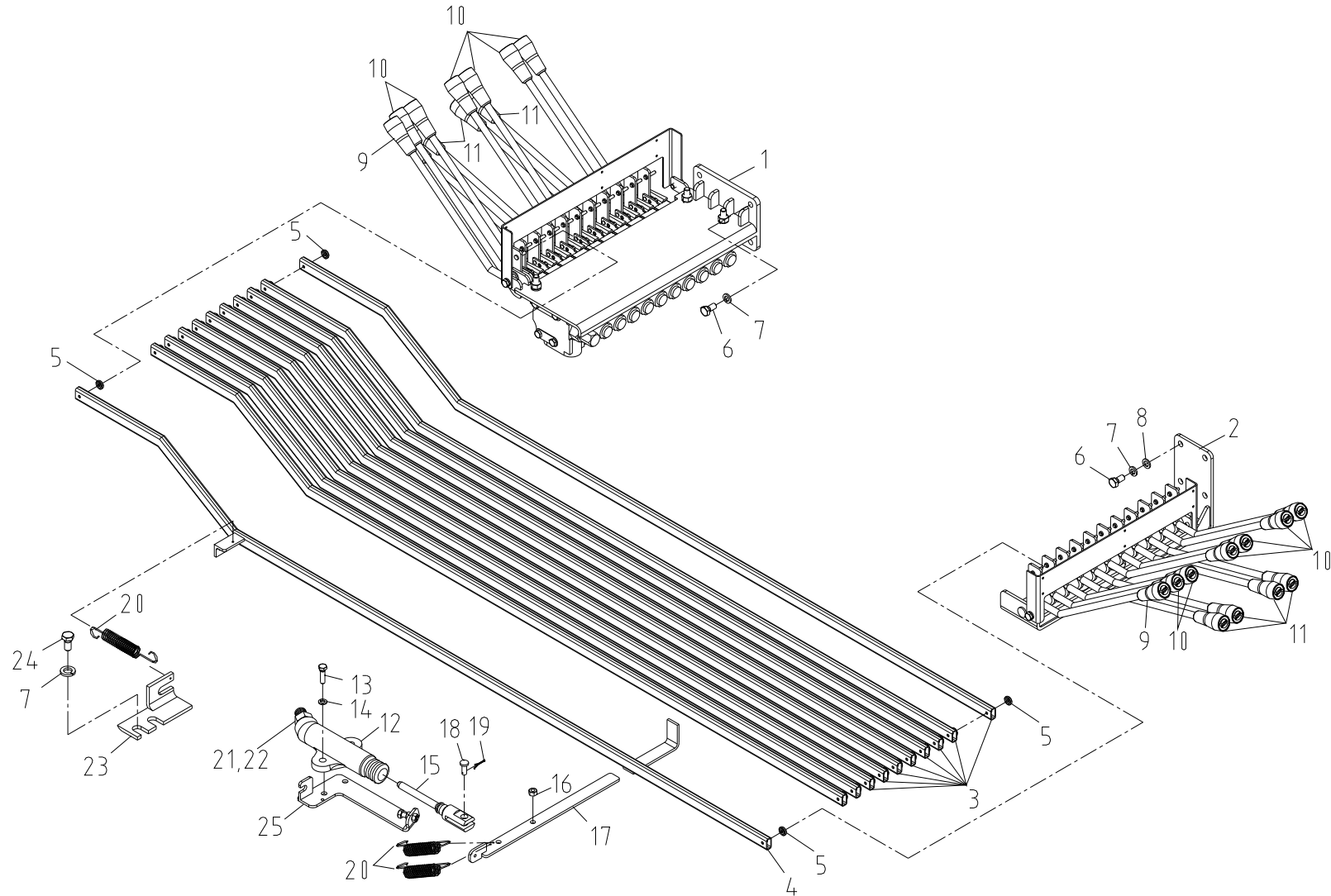
오퍼레이션 조립체 Fig. 3-2 SCS1516L OPERATION ASS'Y
