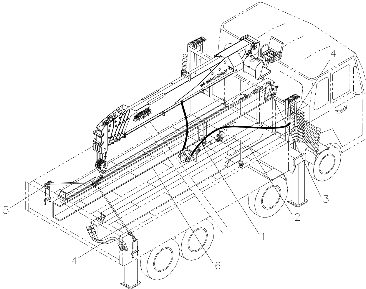
장착 조립체 Fig. 9 SCS1516L MOUNTING ASS'Y
