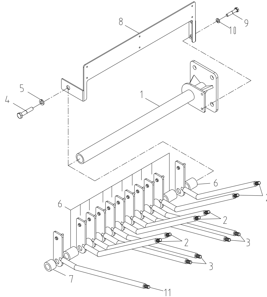
레버 스텐드 세트 Fig. 3-2-2 SCS1516L LEVER STAND SET
