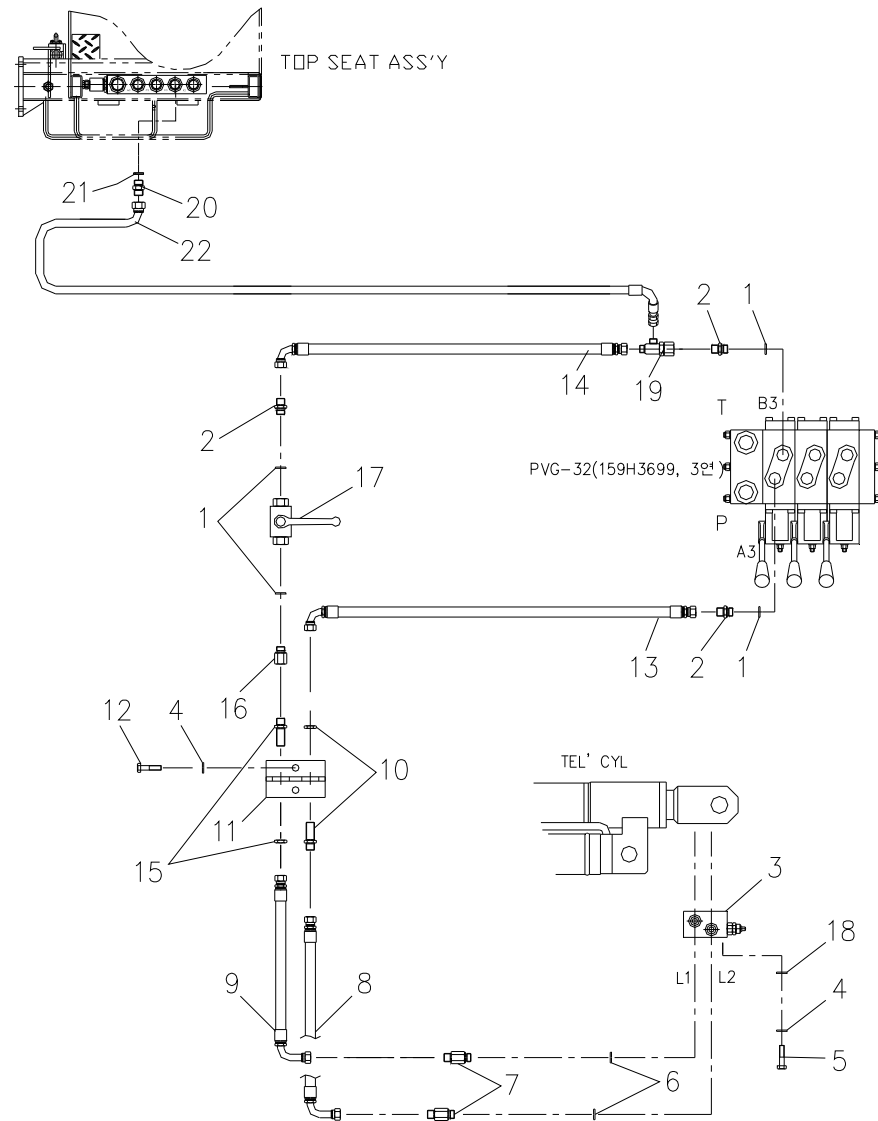
텔레스코픽 배관 Fig. 5-4 SCS1516L TELESCOPIC PIPING
