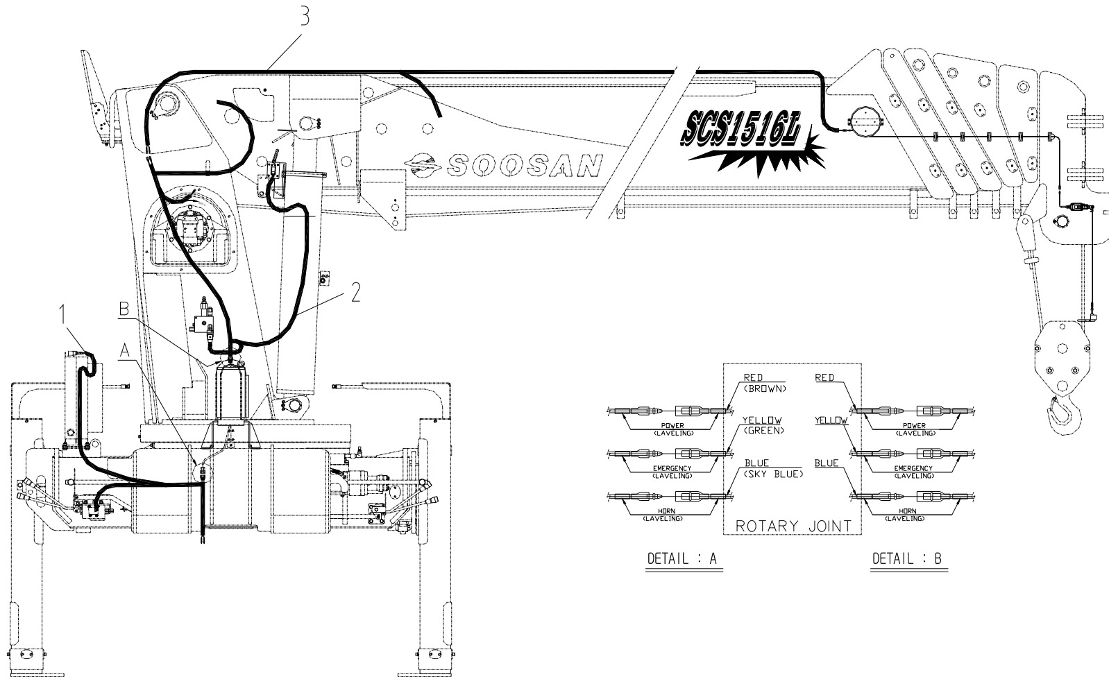
전선 조립체 Fig. 10 SCS1516L WIRING ASS'Y
