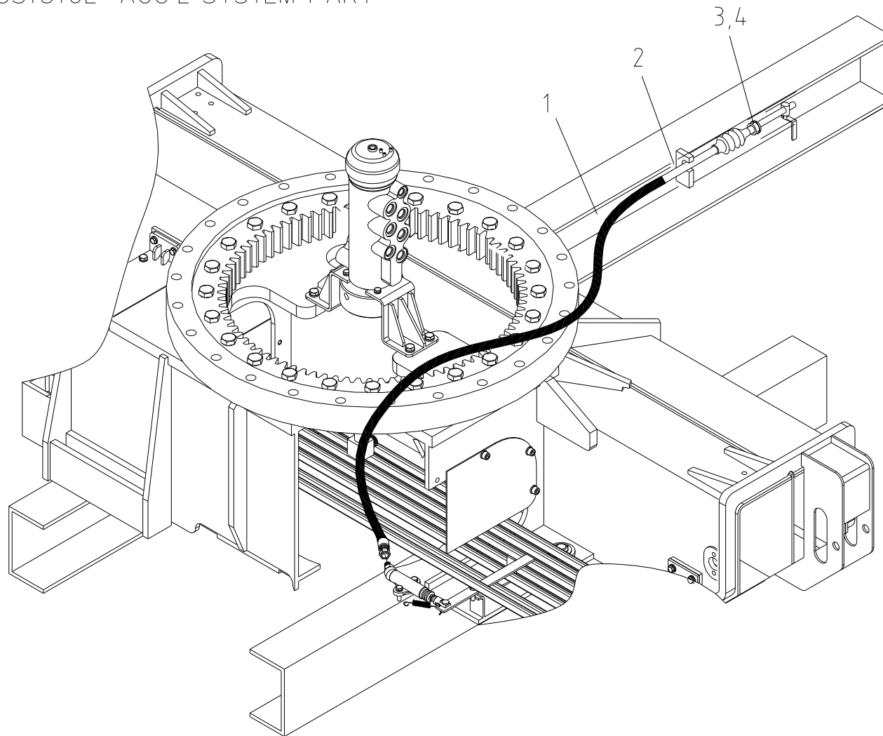
악셀 시스템 파트 Fig. 9-3 SCS1516L ACC'L SYSTEM PART
