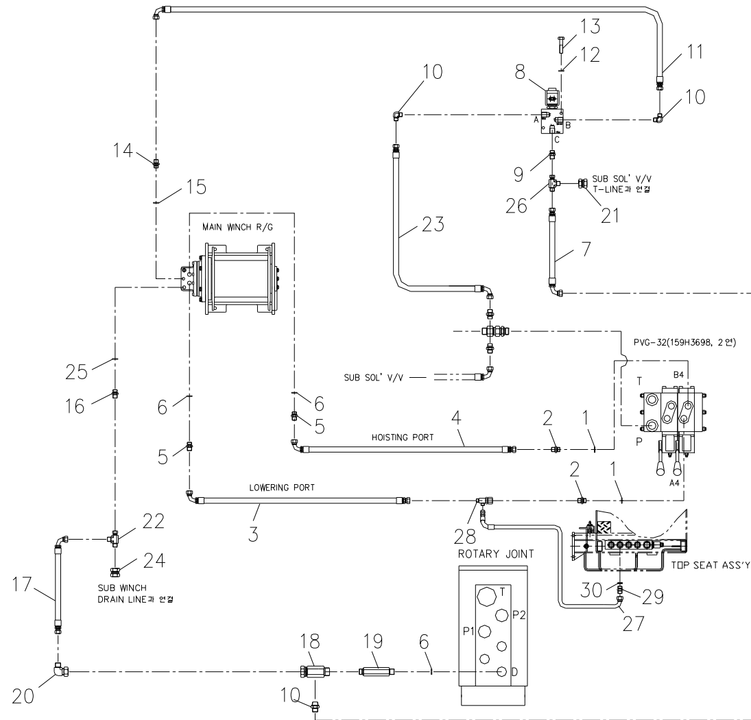
메인 윈치 배관 Fig. 5-5 SCS1516L MAIN WINCH PIPING
