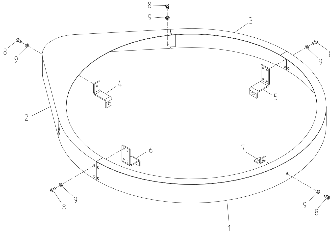
기어 커버 세트 Fig. 3-3 SCS1516L GEAR COVER SET
