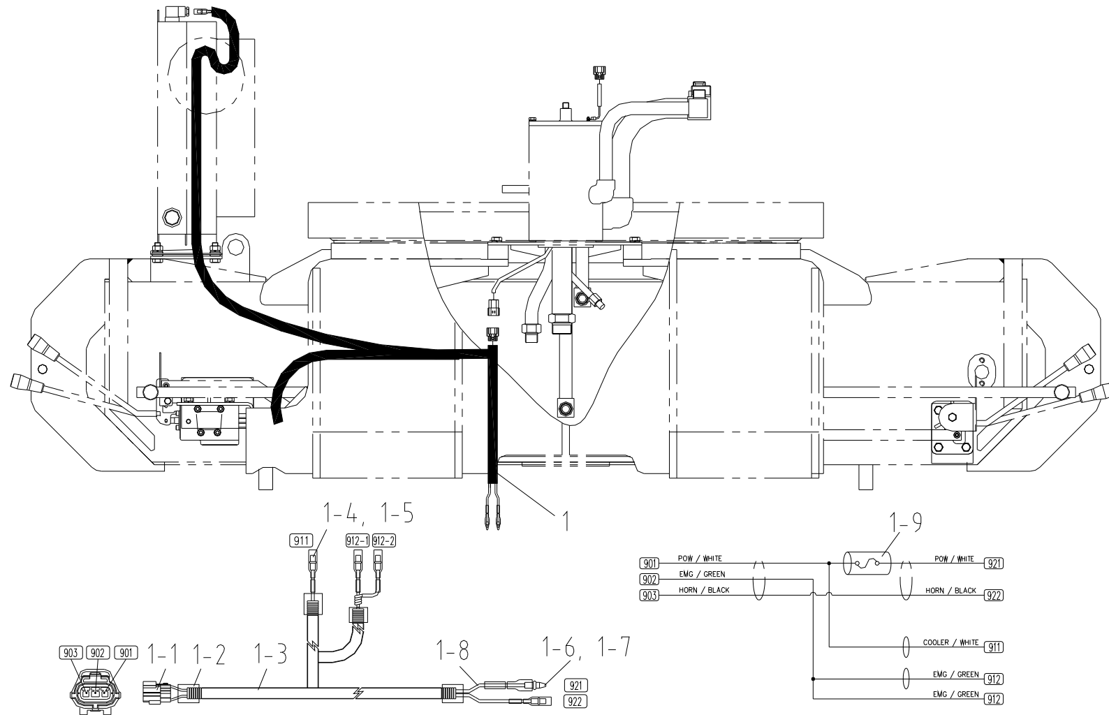
프레임 전선 Fig. 10-1 SCS1516L FRAME WIRING
