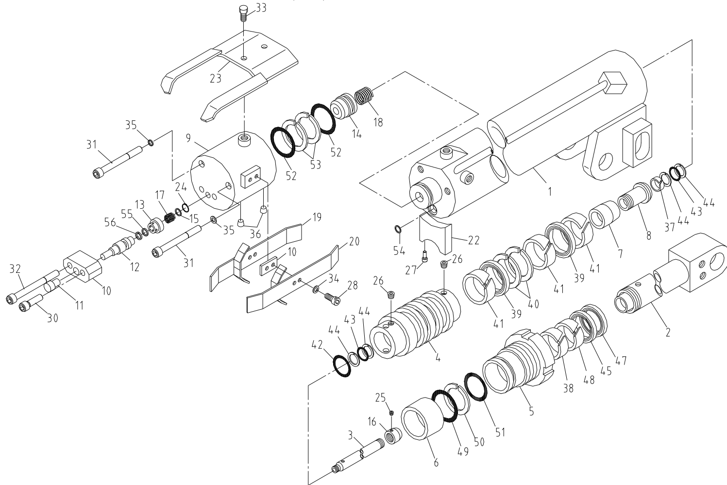
텔레스코픽 실린더(1단) 조립체 Fig. 1-1-1 SCS1516L TELESCOPIC CYL'(1st) ASS'Y
