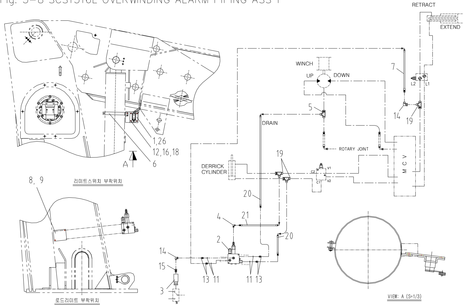
과하중 방지 배관 조립체 Fig. 5-8 SCS1516L OVERWINDING ALARM PIPING ASS'Y
