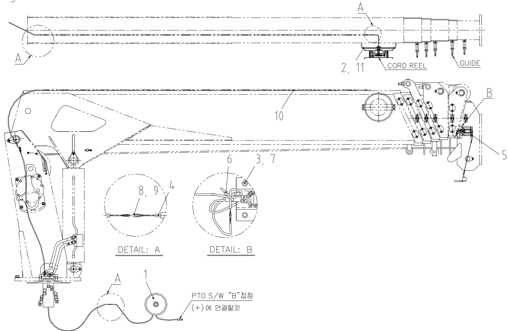
Fig. 15 과권방지장치 조립체
