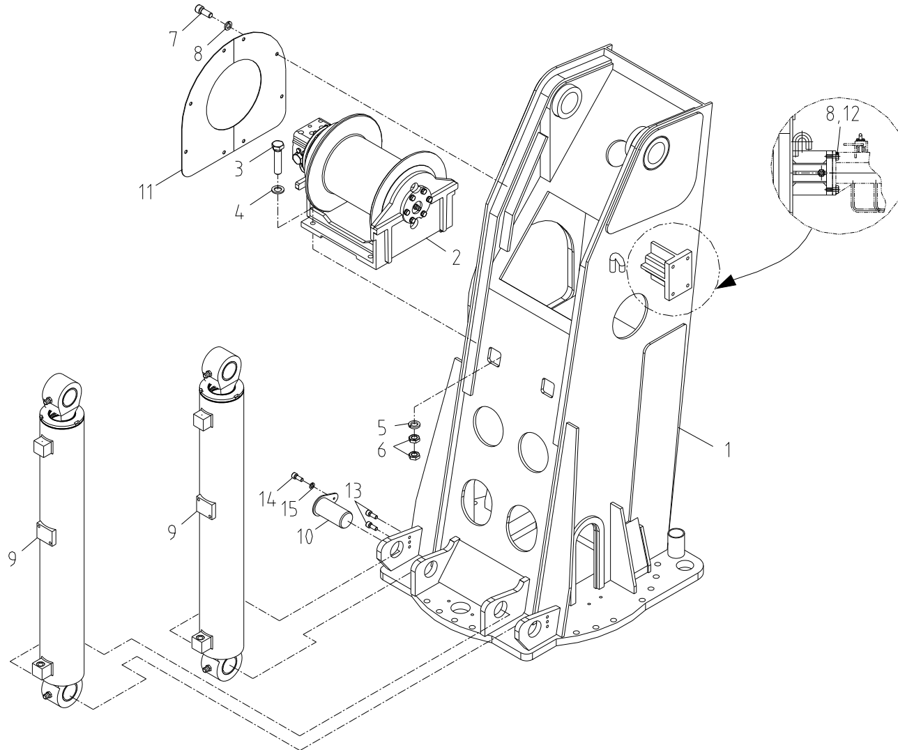
스윙 포스트 조립체 Fig. 2 SCS1516L SWING POST ASS'Y
