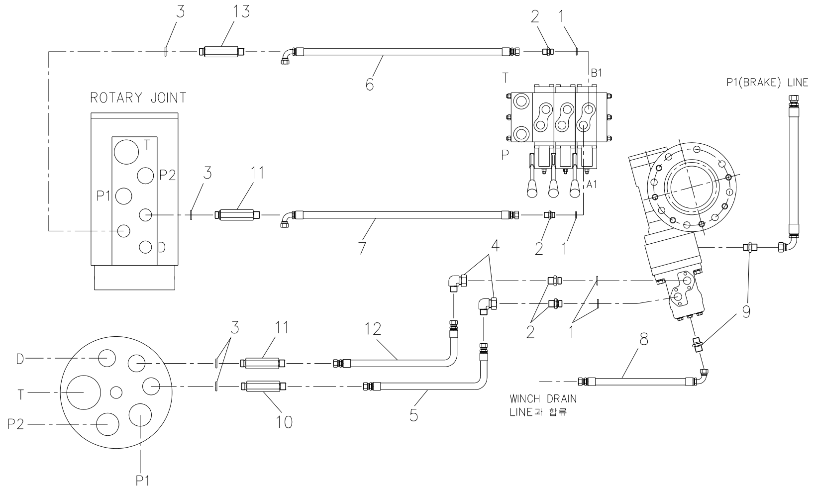
스윙 배관 Fig. 5-2 SCS1516L SWING PIPING
