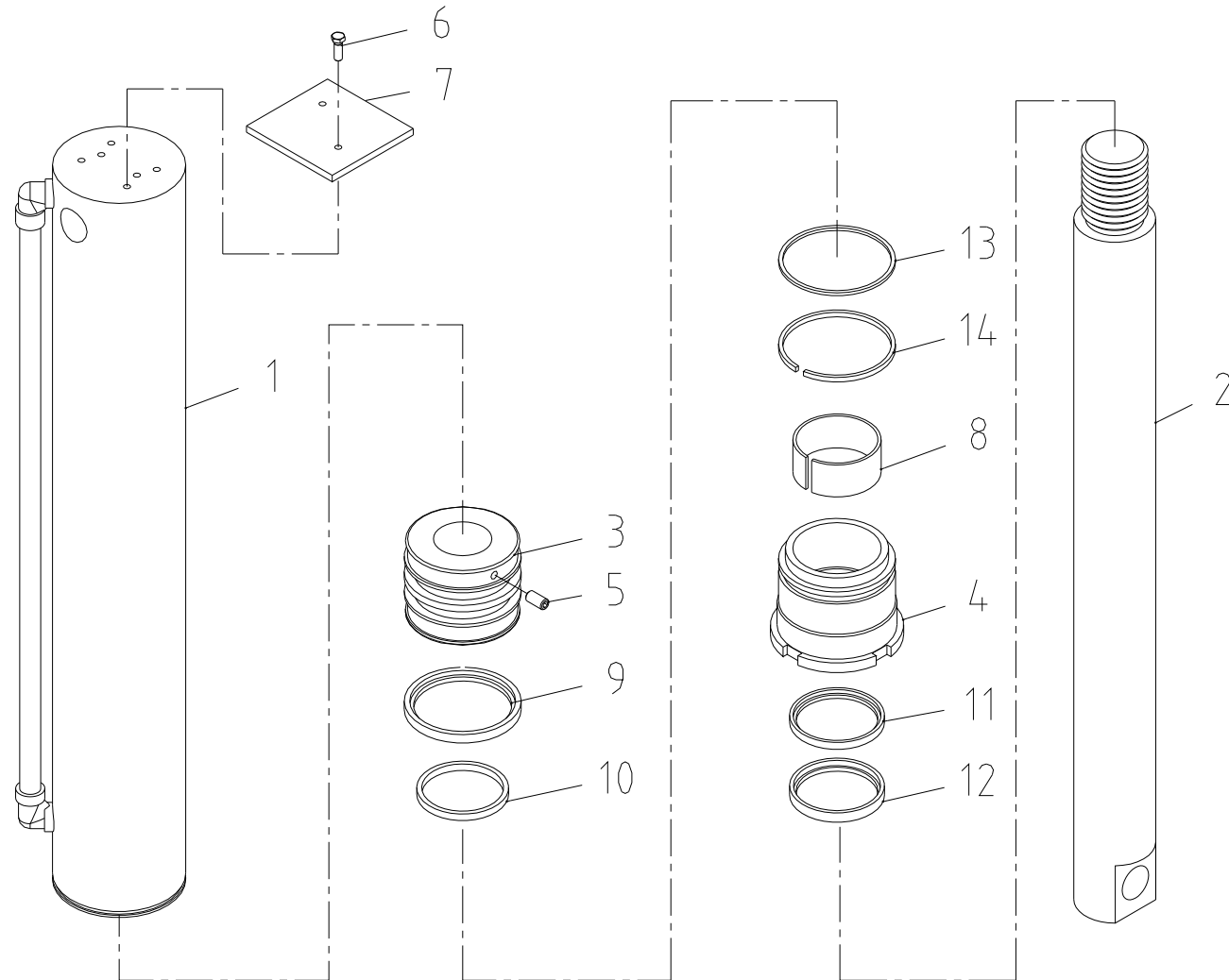
잭 실린더 조립체 Fig. 9-2-1-1 SCS1516L JACK CYL' ASS'Y
