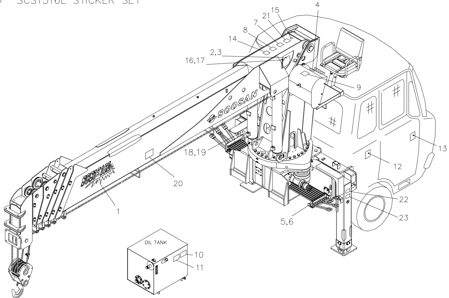
스티커 세트 Fig. 7 SCS1516L STICKER SET
